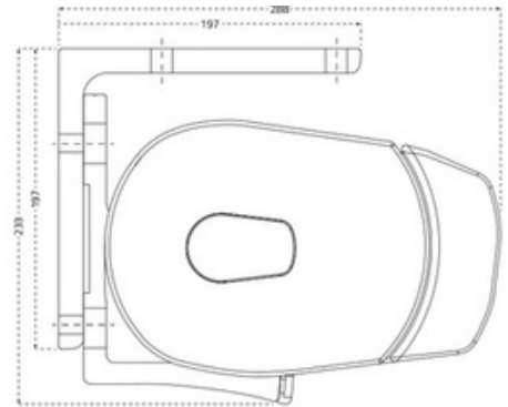
Plafondmontage
